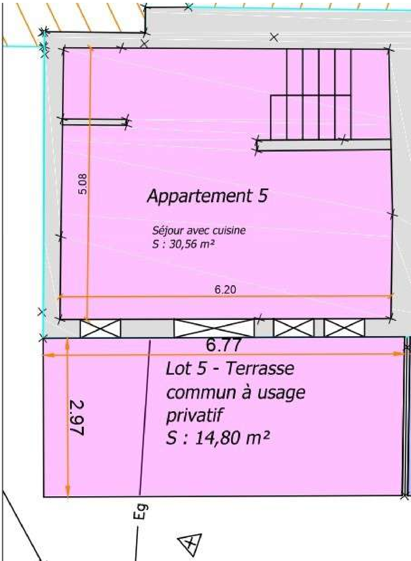
PLAN rez-de-chaussée - 1/100
