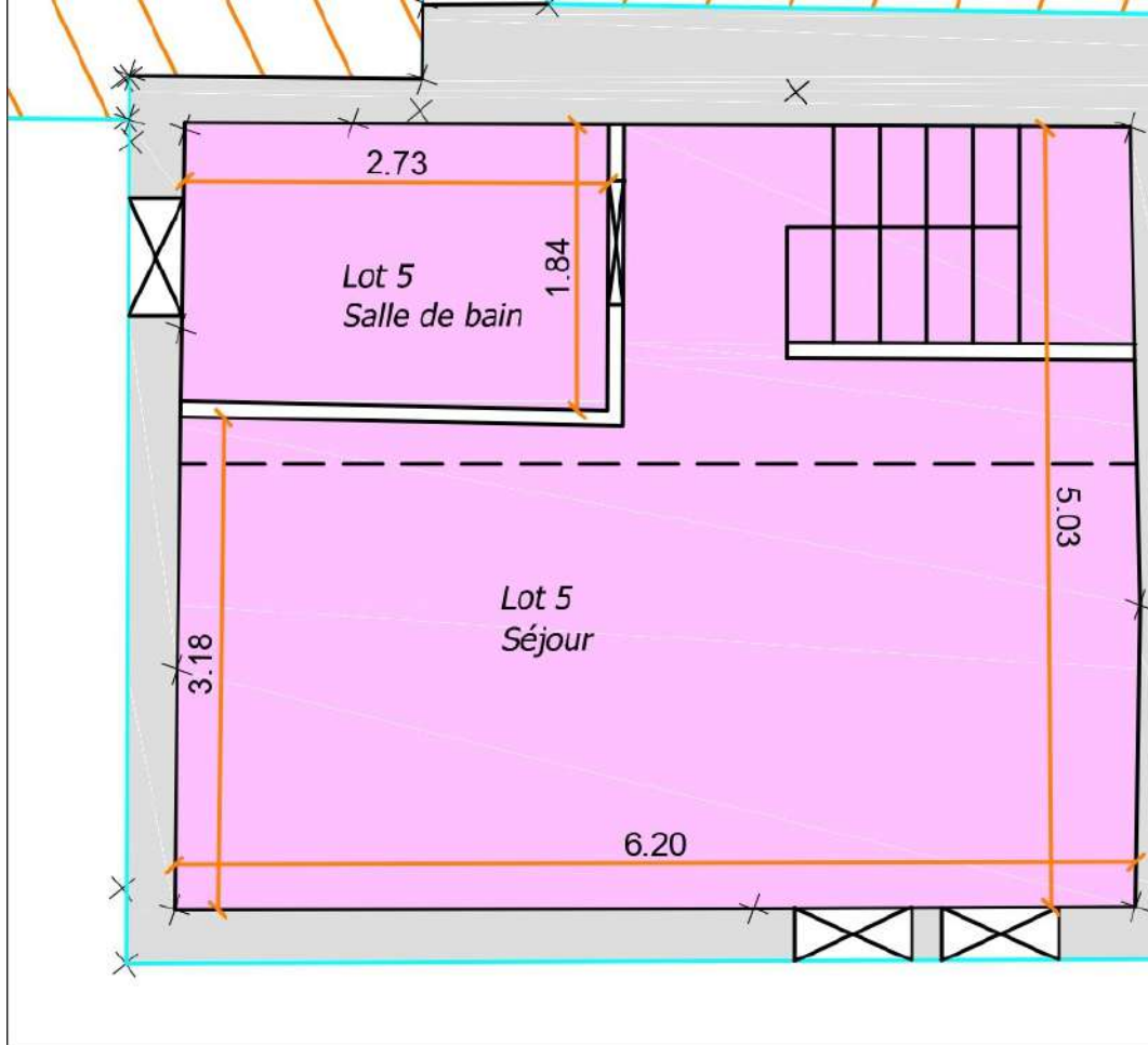
PLAN 1er étage - 1/100
